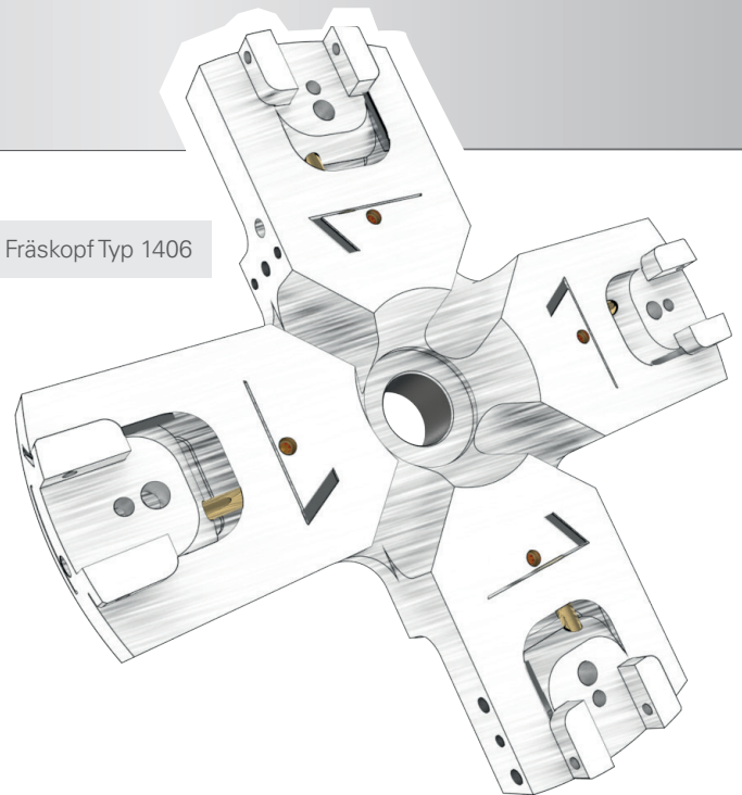
Fräskopf für das Planfräsen
